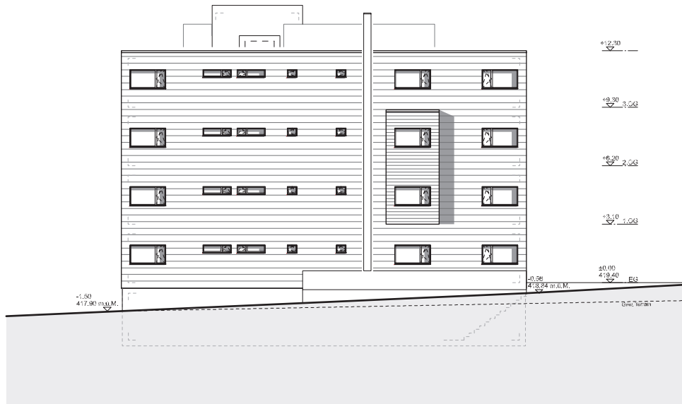
Nordfassade
