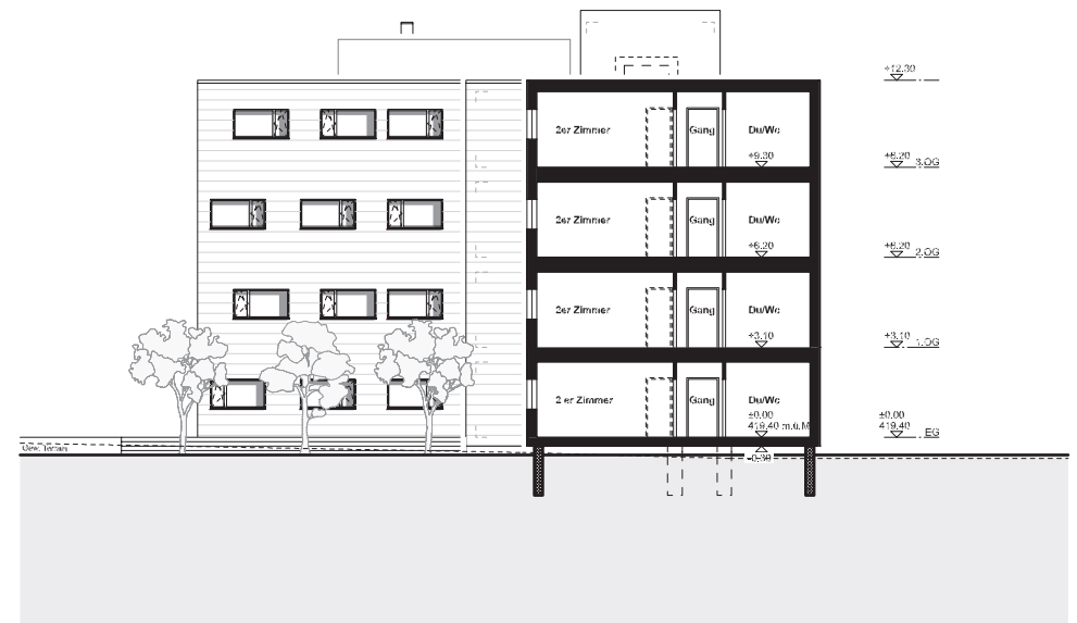
Schnitt B-B
