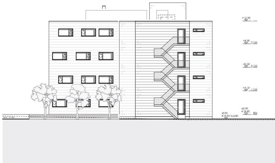
Südfassade
