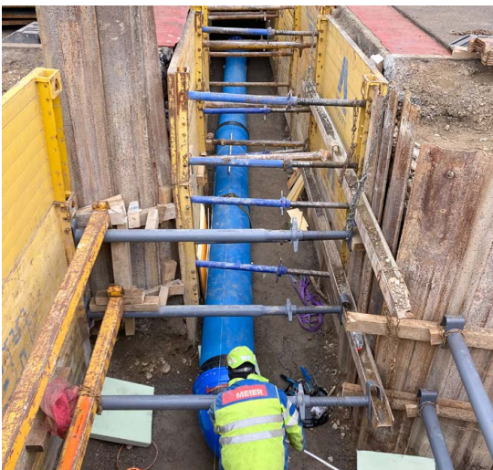
47 Umlegung Wassertransportleitung
