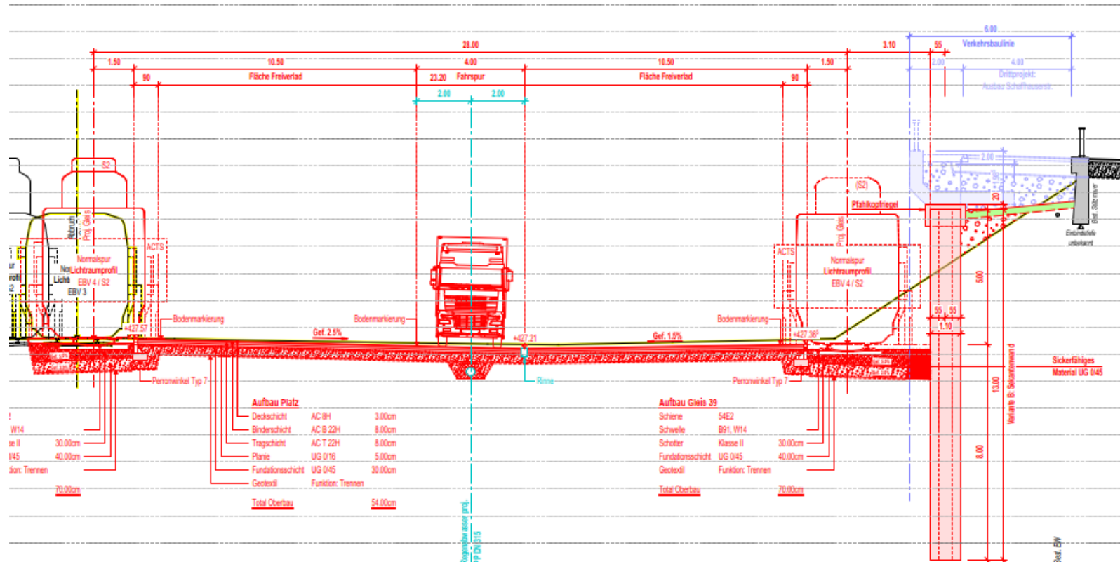
Ausschnitt Querprofil Stützbauwerk.
