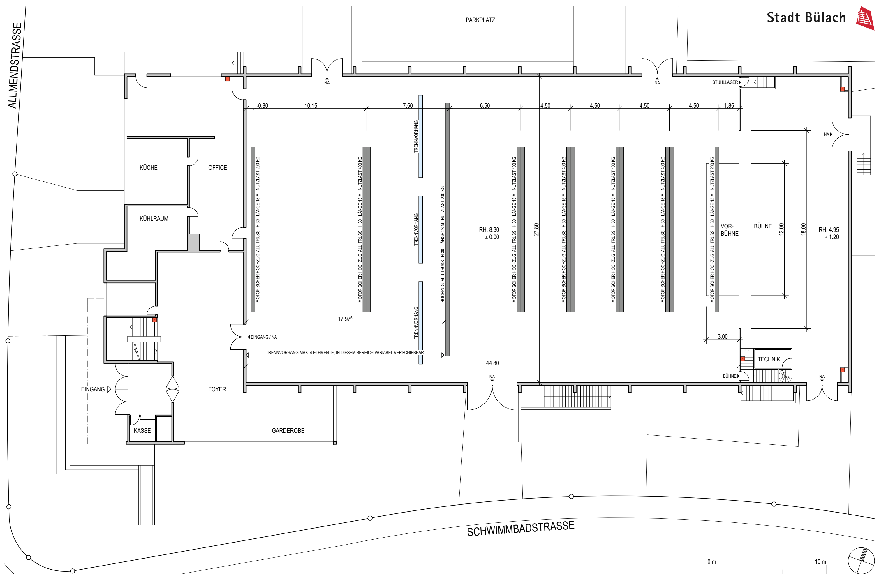
TECHNISCHER PLAN
