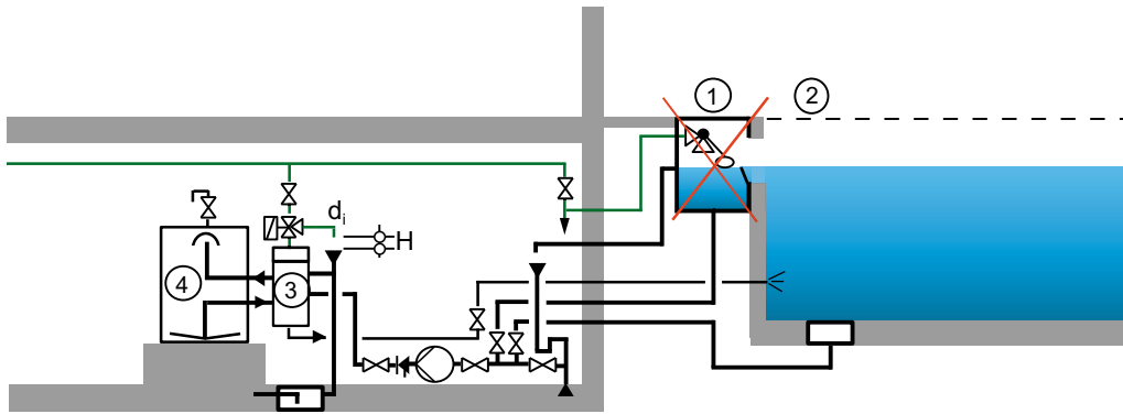
Abb. 1 Private Badeanlage mit Skimmer
