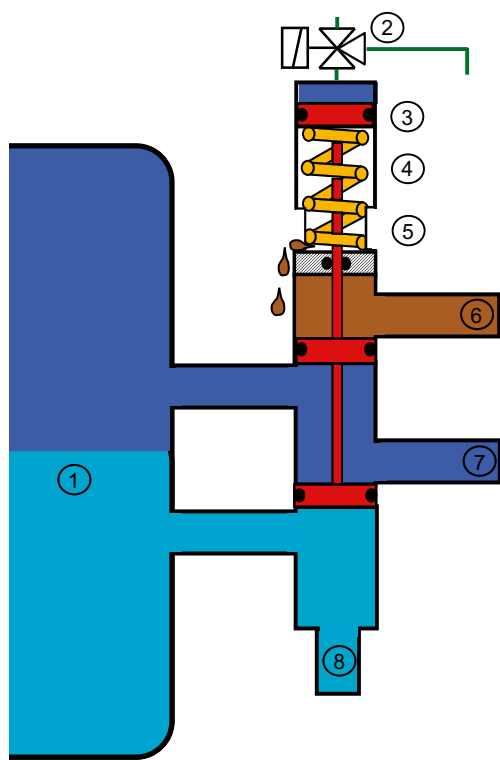
Abb. 16 Detail Antriebsgehäuse
