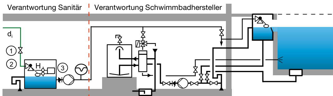
Abb. 7 Private Badeanlage mit freiem Auslauf Bauart AB
