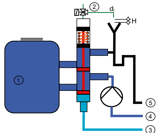
Abb. 15 Rückspülung
