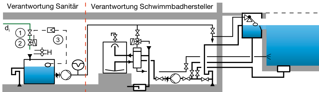
Abb. 6 Private Badeanlage mit freiem Auslauf Bauart AA
