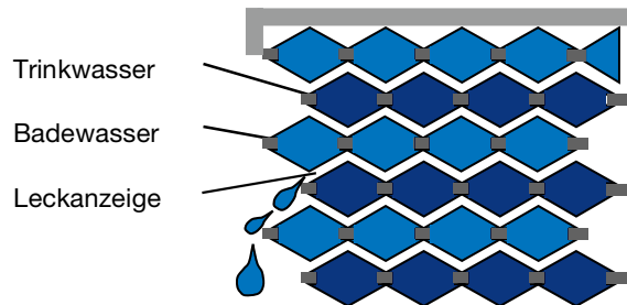
Abb. 13 Schnitt durch Plattentauscher
