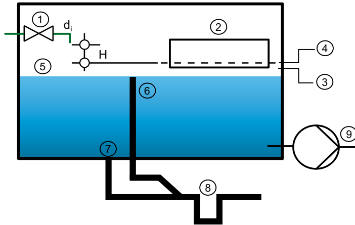
Abb. 3 Freier Auslauf Bauart AB
