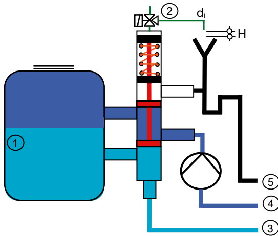
Abb. 14 Betriebsstellung
