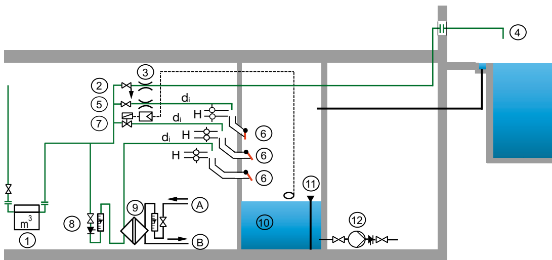
Abb. 10 Badeanlage mit Ausgleichsbecken
